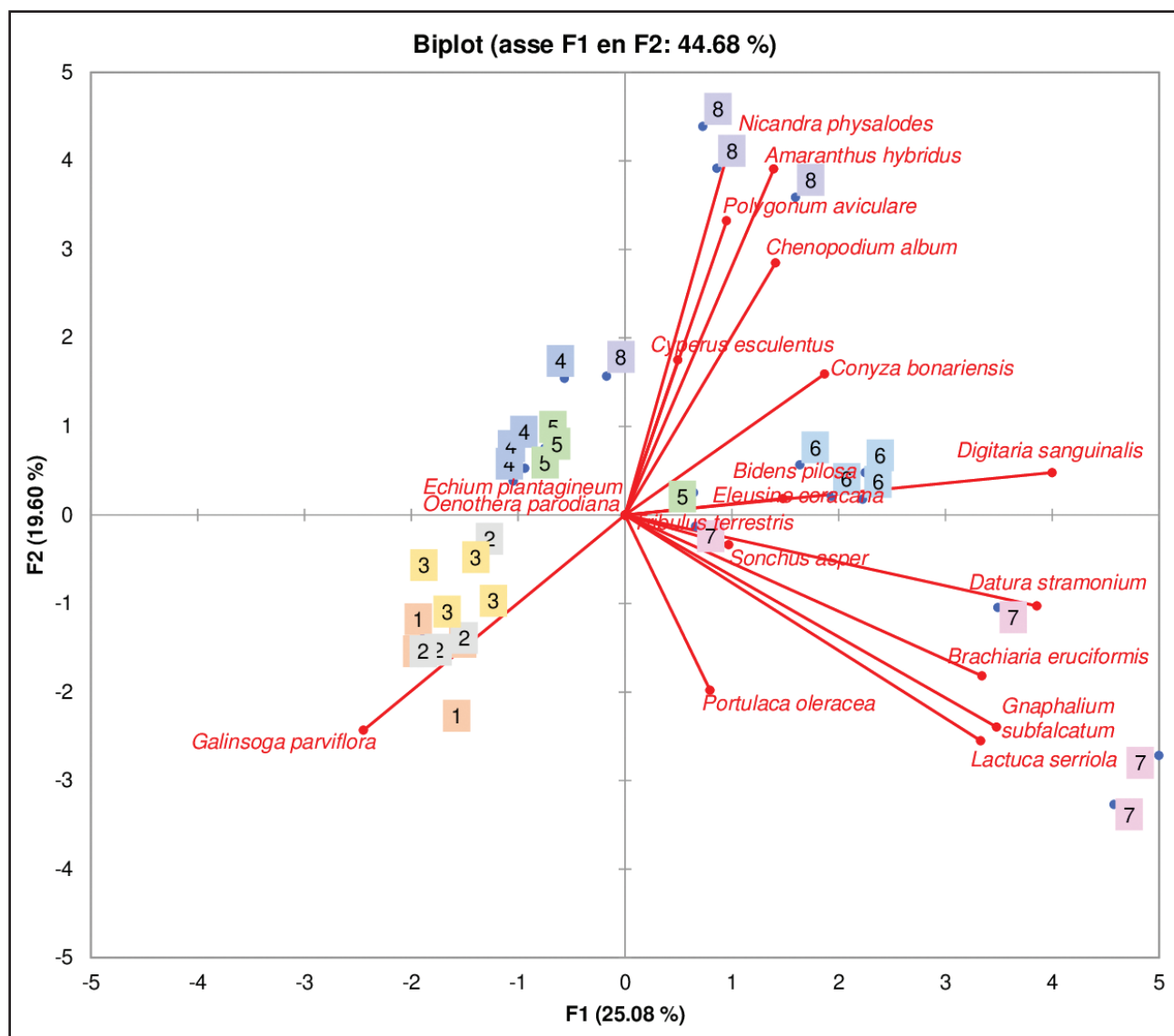
FIGUUR 1: Tellinggrafiek van die populasi-samestelling van someronkruidspesies se finale spektrum op George, en die assosiasies daarvan met smoorgewasverbuigings-praktyke wat aangedui word deur die Behandelingnummers 1-8.
